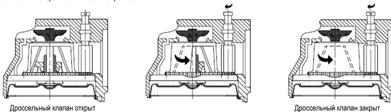
Рис. 7. Настройка дроссельного клапана
