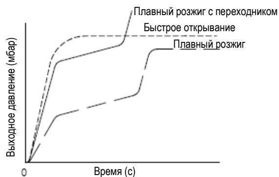
Рис. 5. Характеристики открывания
