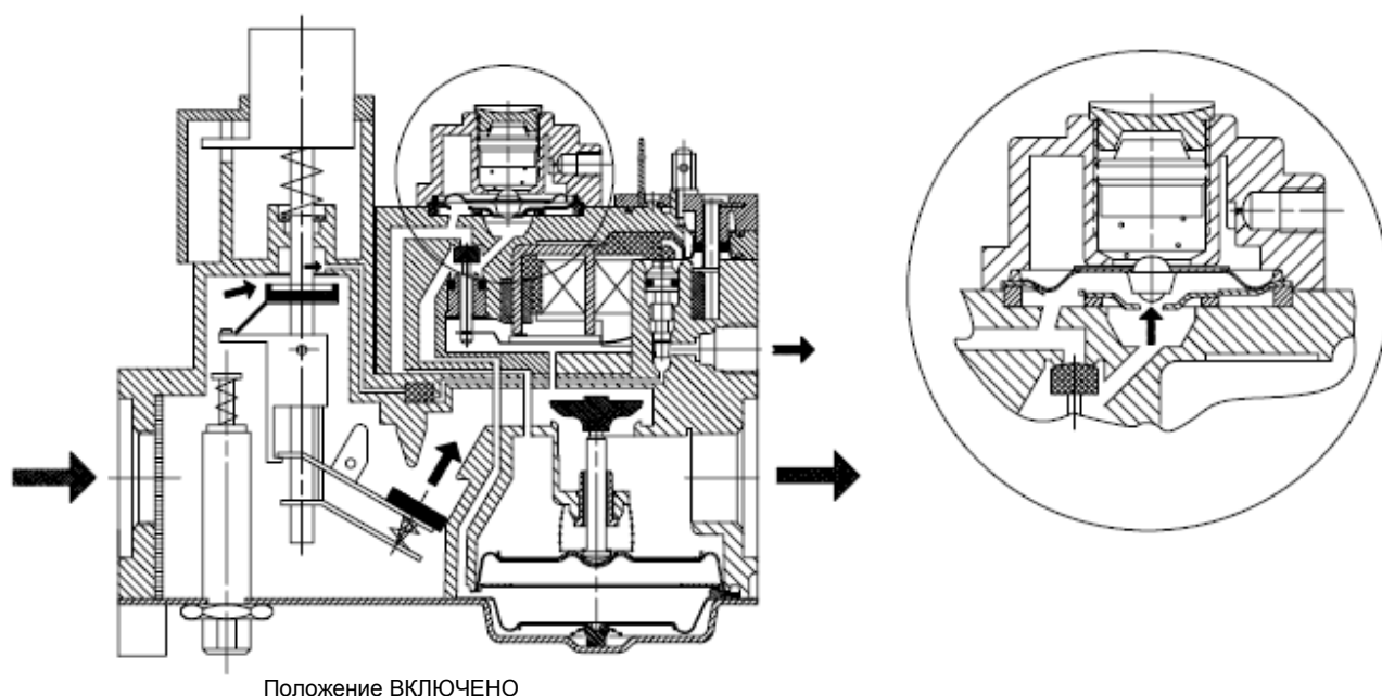
Рис. 4. Серворегулирование давления
